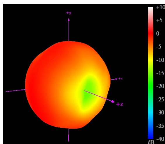
2450MHz
