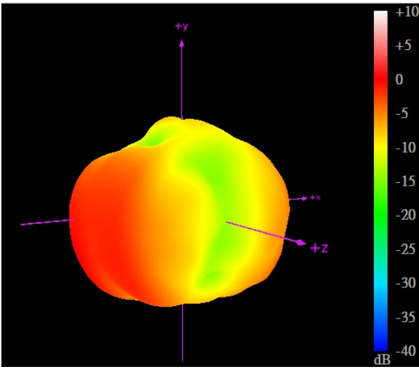
2500MHz
