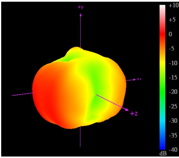
2540MHz
