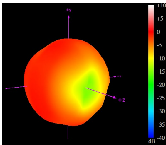
2500MHz
