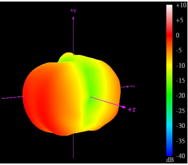
2400MHz
